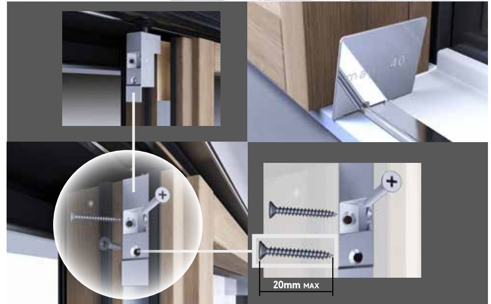
8 | Montaggio dell'anta scorrevole e degli accessori Assembly of the sliding sash and the accessories
