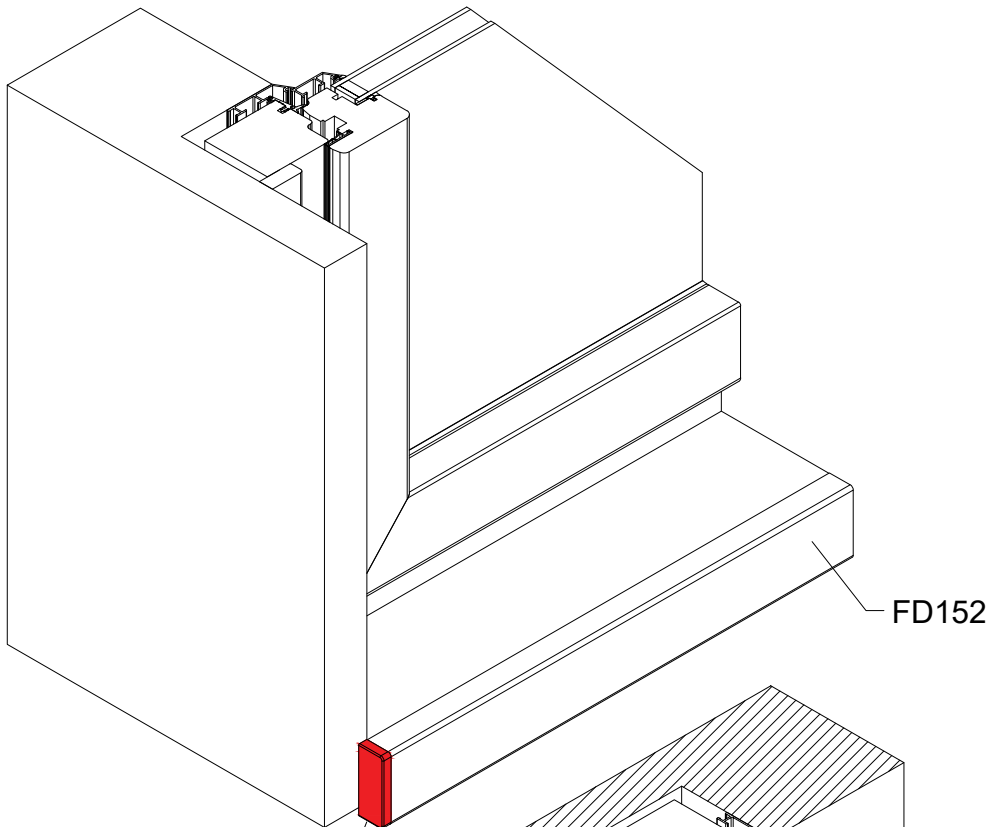
Terminale laterale LC61/70A
