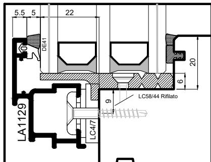
A4: LA1129/battuta 20mm
