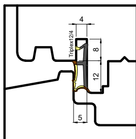
B2: Guarnizione su anta
