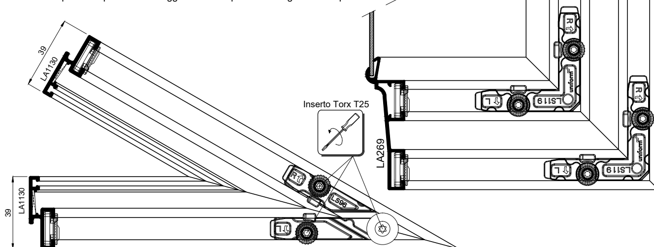
LS99: Squadretta per l'assemblaggio a vite dei profili con angolo fuori squadra
