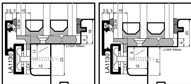
A3: LA1129/battuta 18mm
