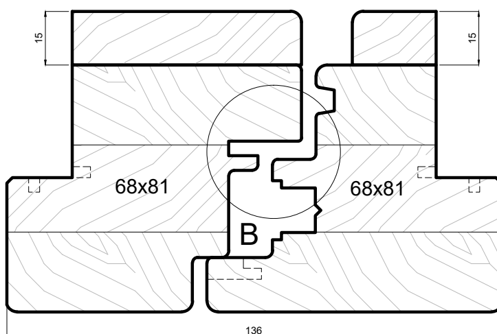
B2: Guarnizione su anta
