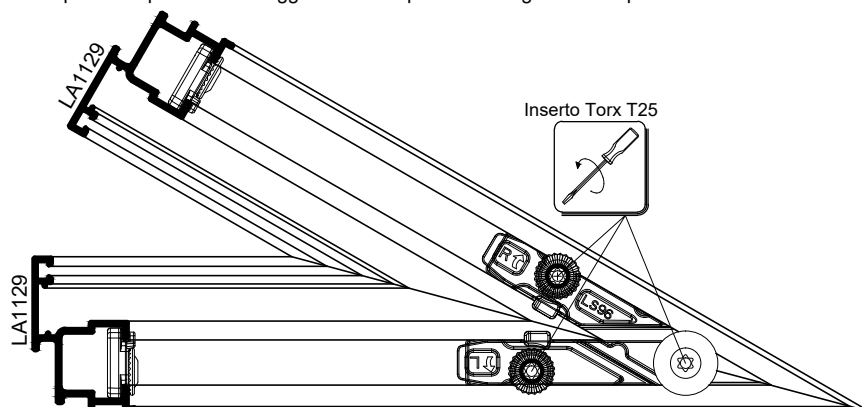
LS96: Squadretta per l'assemblaggio a vite dei profili con angolo fuori squadra
