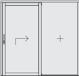
Alzante scorrevole con un'anta scorrevole e vetro laterale fisso Single sash lift & slide door with side fixed light frame
