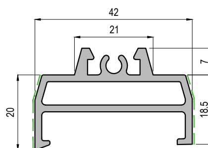
PA251 Binario per alzante scorrevole Rail
