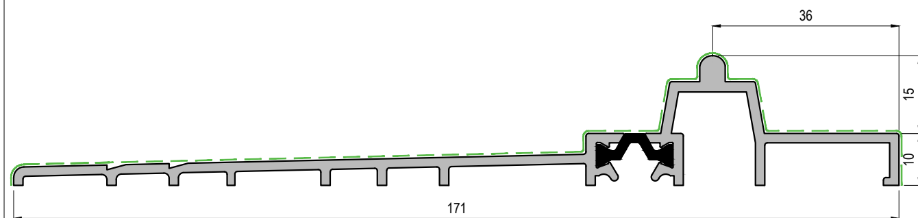
PA135T Soglia in alluminio a taglio termico Aluminium Treshold
