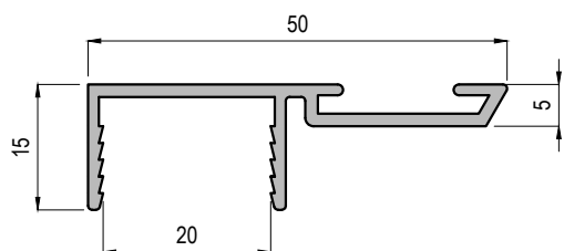
PA95 PA95C - Con lavorazione di zancatura
