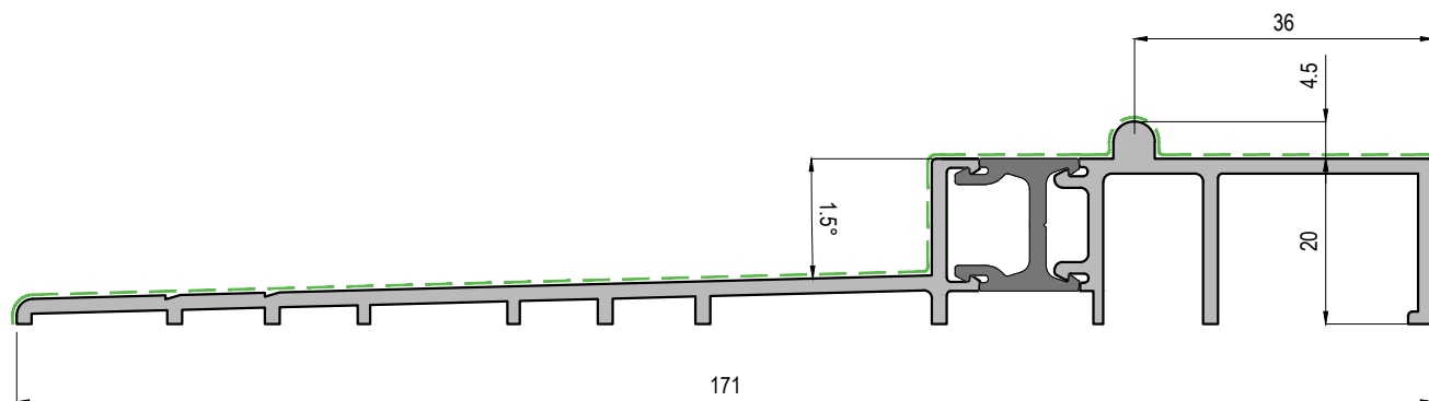
PA249T Soglia in alluminio a taglio termico Aluminium Treshold
