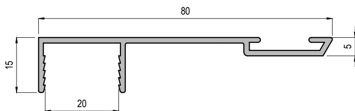
PA97 PA97C - Con lavorazione di zancatura
